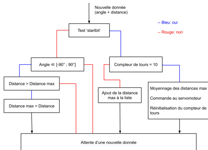
Figure 5 - Schéma de fonctionnement l'algorithme de traitement de données du lidar
