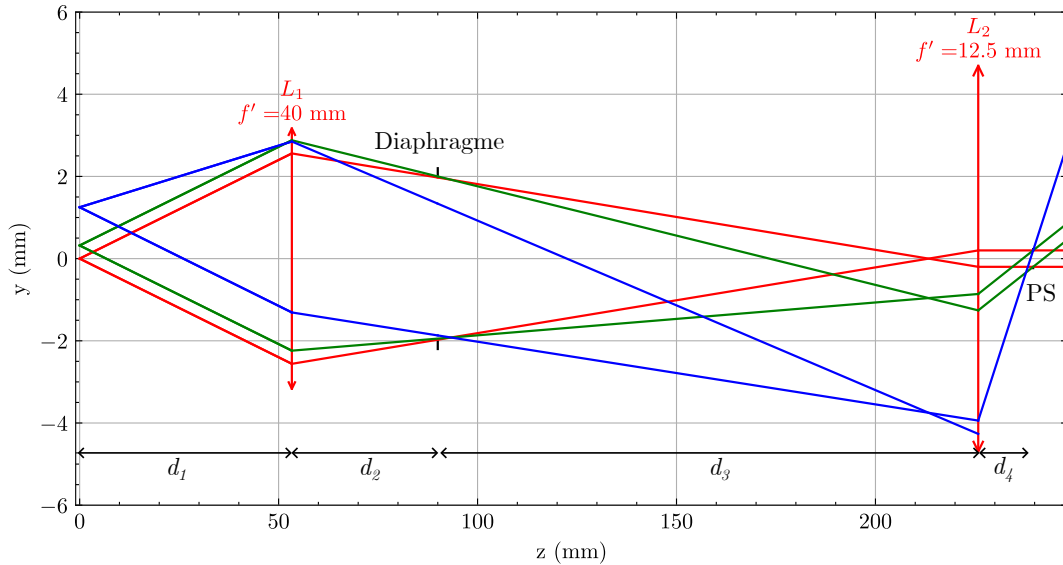
Figure 2. Schéma du microscope du TD d'Optique Instrumentale.
